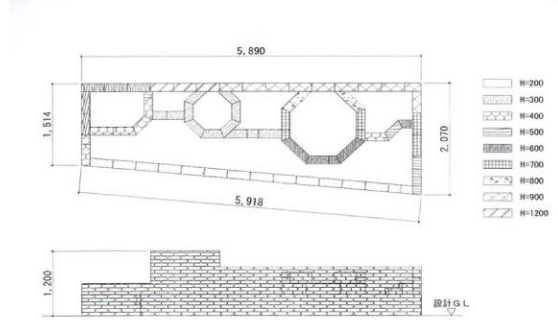
カルセラタイル花壇詳細図 1/50
